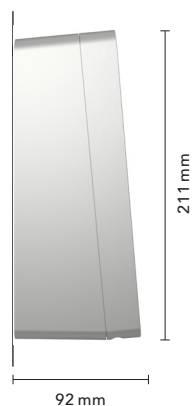
Wandmontage (HD-Box)
